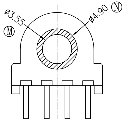
SEC.A-A
